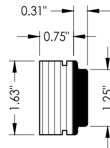
HINGE & LATCH STILE
